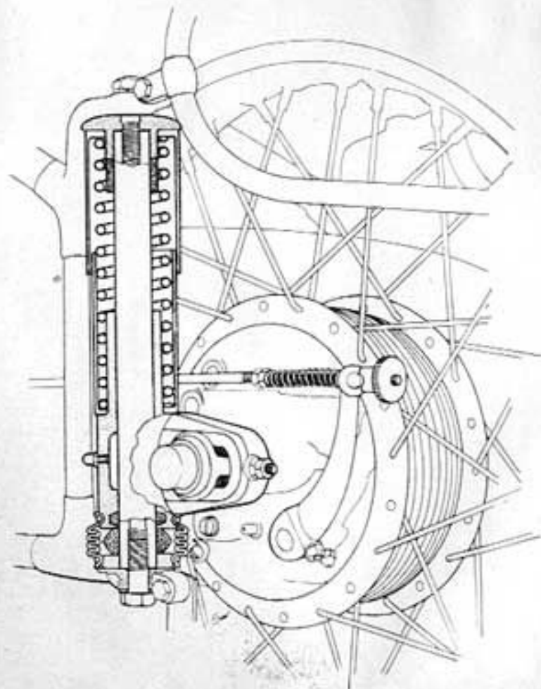
Schnittbild der Hinterrad-Federung
