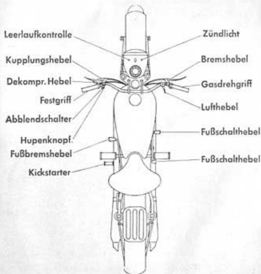
Ansicht des Motorrades mit Bedienungshebeln
