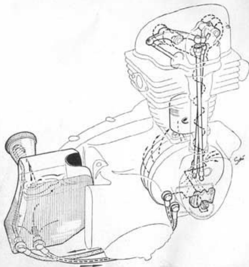
Trockensumpf-Umlaufschmierung
