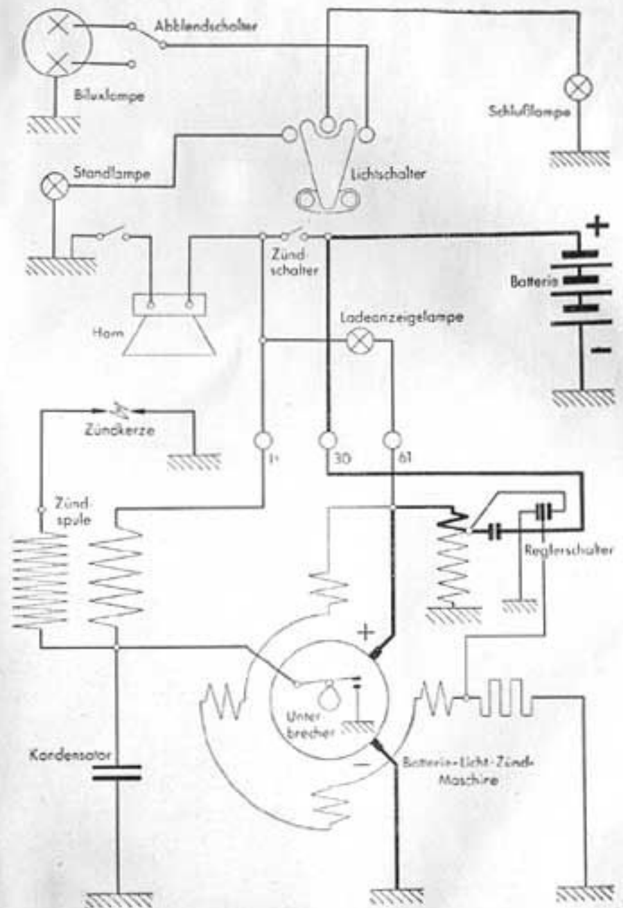
Inneres Schaltbild der HOREX „Regina“ Batterie-Lichtzünd-Anlage
