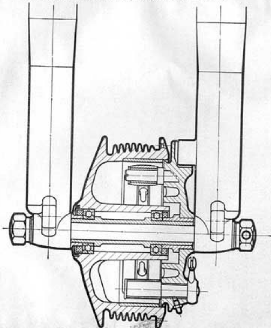
Schnittbild der Vorderrad-Bremsnabe
