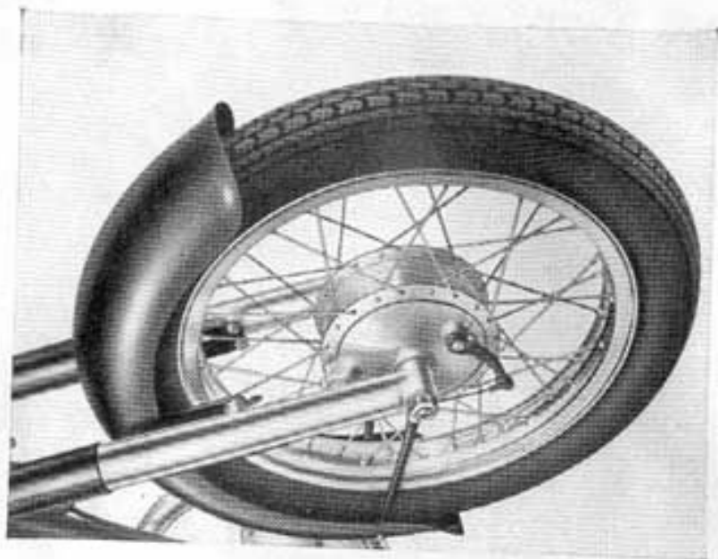
Vorderrad-Bremsnabe
