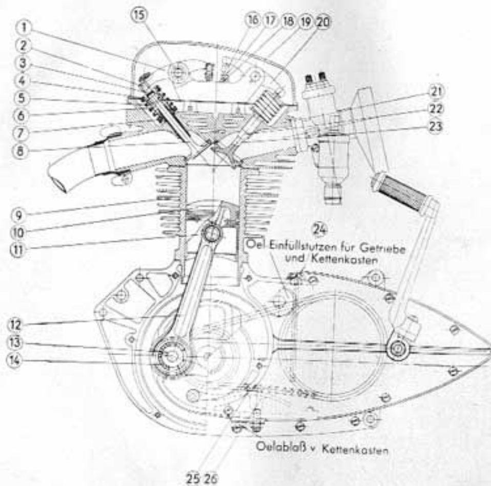
Schnittbild des Motors (Antriebsseite)
