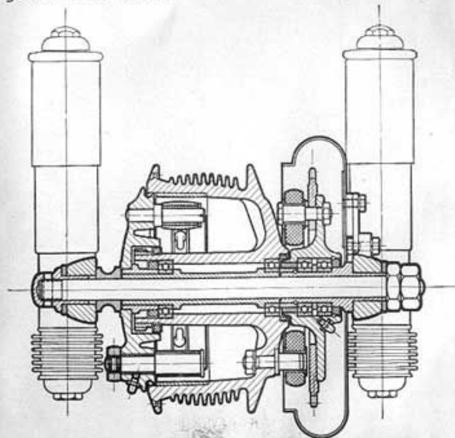
Schnittbild der Hinterrad-Bremsnabe
