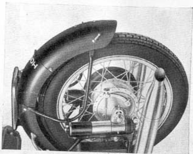
Hinterrad-Bremsnabe
